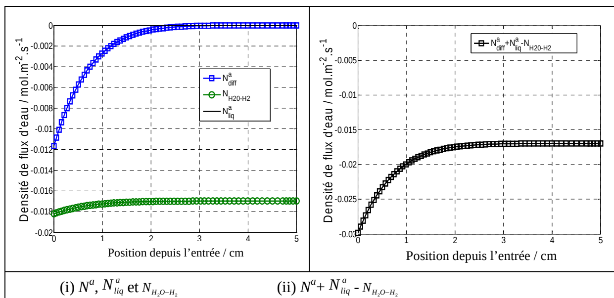
Figure 5.24 Différents flux d'eau traversant la couche poreuse côté anode en fonction de la longueur du canal pour T_a > T_c avec D_m = 1.9 \text{ m}^2.\text{s}^{-1} et \xi = 0.55 à j = 1.4 \text{ A.cm}^{-2}
