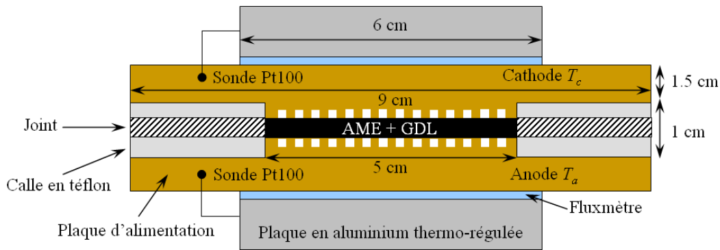
Figure 3.15 Schéma de principe du montage des fluxmètres
