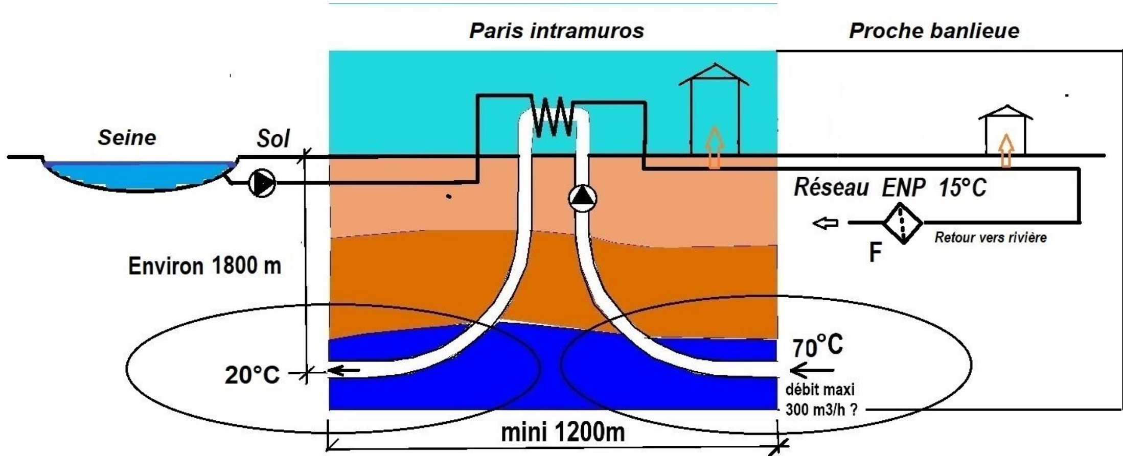
Figure 36 se reporter à la figure 34 précédente pour compréhension du transfert thermique
