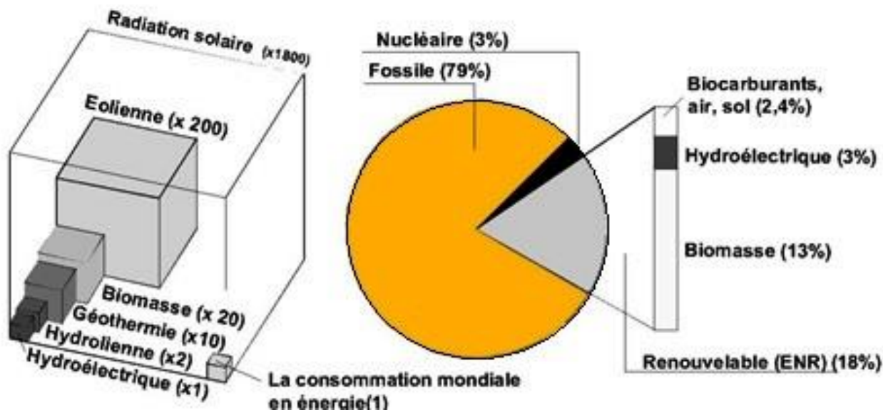
Figure 1 Valeurs IRENA
